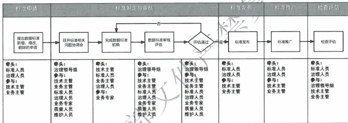
图2 数据标准管理流程图
